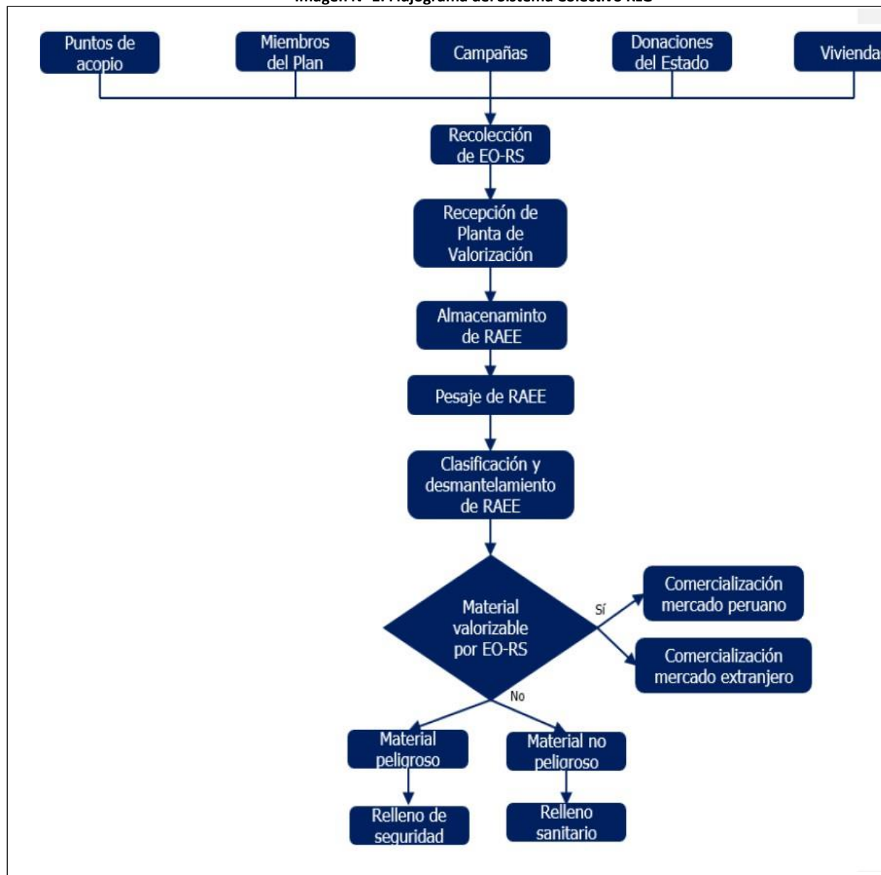
Imagen N° 1: Flujograma del Sistema Colectivo RLG
